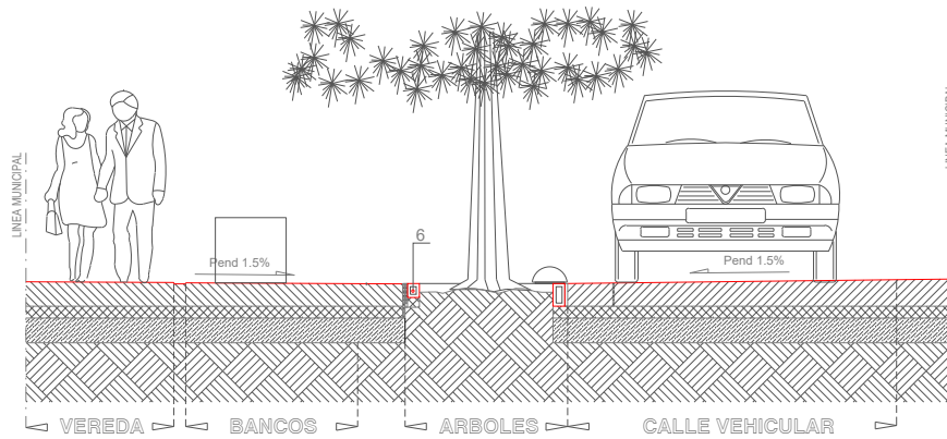
SECCIONESQUEMATICA3-3
