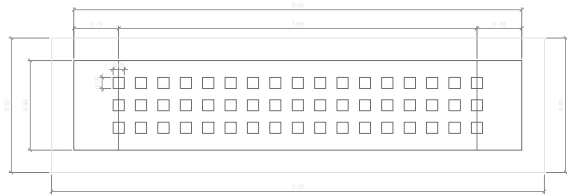
Corte - Vista Frente
