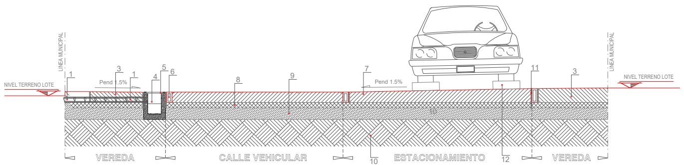
SECCIONESQUEMATICA2-2
