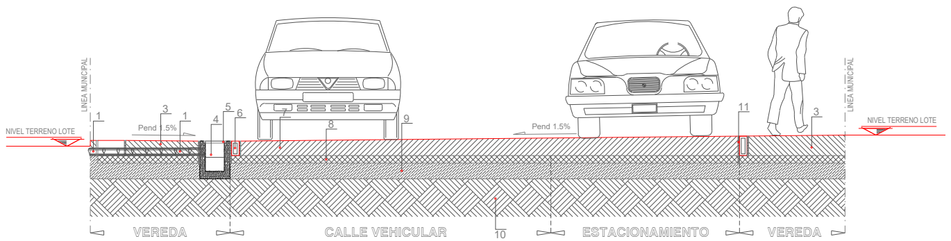
SECCIONESQUEMATICA1-1
