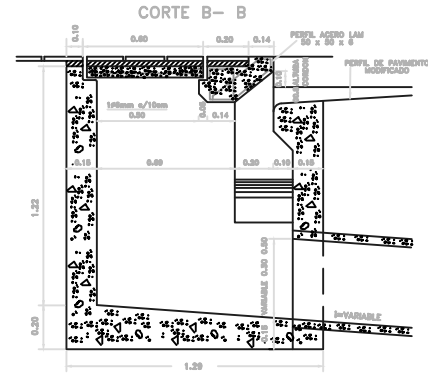
VARIANTE CON CAÑO DE SALIDA LATERAL
