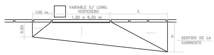
MODIFICACION DE PAVIMENTO PARA FORMACION DE HOYA
