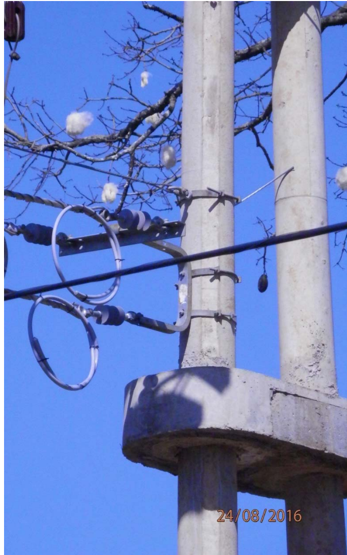
Detalle de la retención con cruzeta metálica tipo C, y aisladores Orgánico
