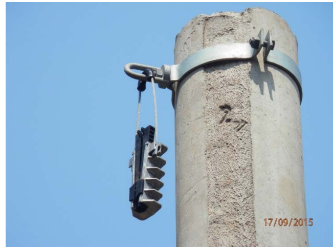
Detalle en la cima abrazadera más pinza de retención PKR10
