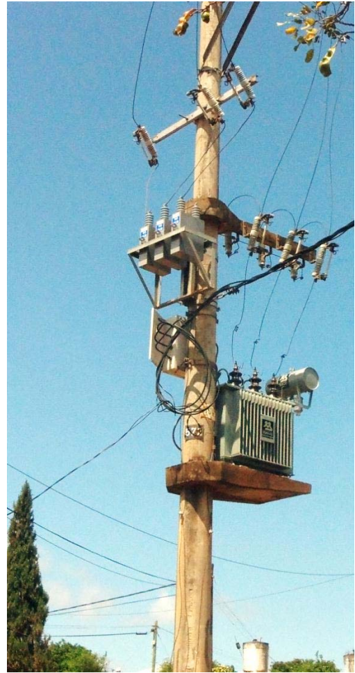
Ubicación posible del banco capacitivo trifásico Para la corrección del factor de potencia
