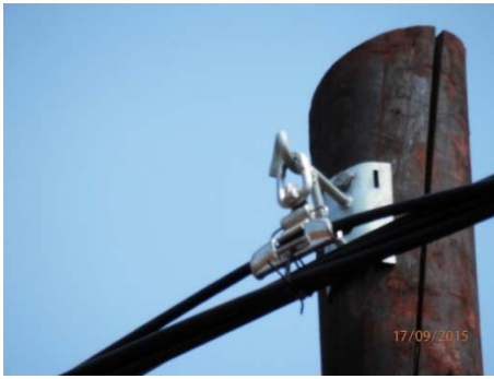
Detalle en la cima de post de madera suspensión simple SSCBN
