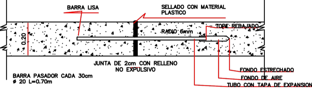
LONGITUDINAL (detalle 3)
