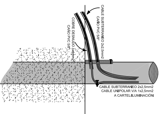
DETALLE ACOMETIDA ELECTRICA
