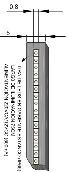
DETALLE ILUMINACIÓN LED
