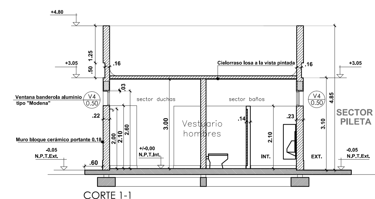
CORTE 1-1
