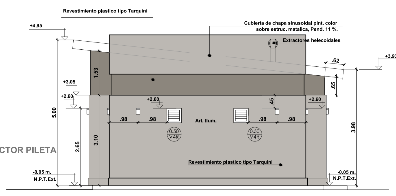
VISTA LATERAL EDIF. VEST. PILETA DESDE VIAS TREN
