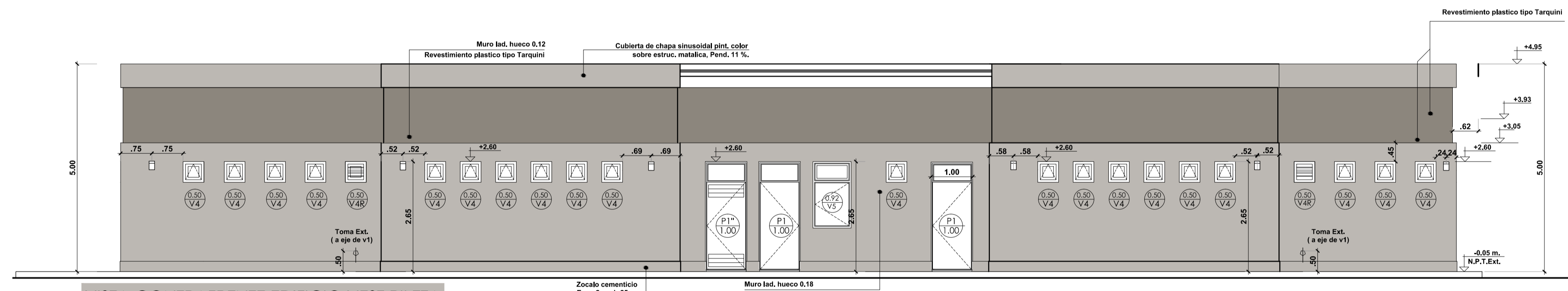
VISTA CONTRAFRENTE EDIFICIO VEST. PILETA DESDE PILETA
