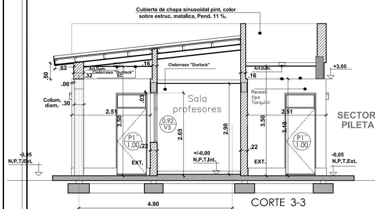
CORTE 3-3
