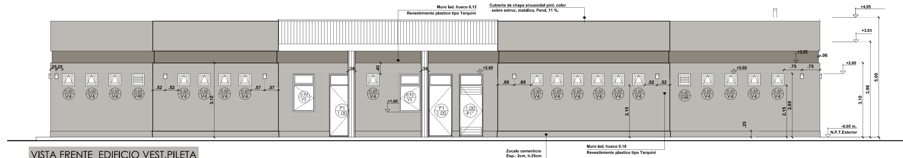
VISTA FRENTE EDIFICIO VEST. PILETA
