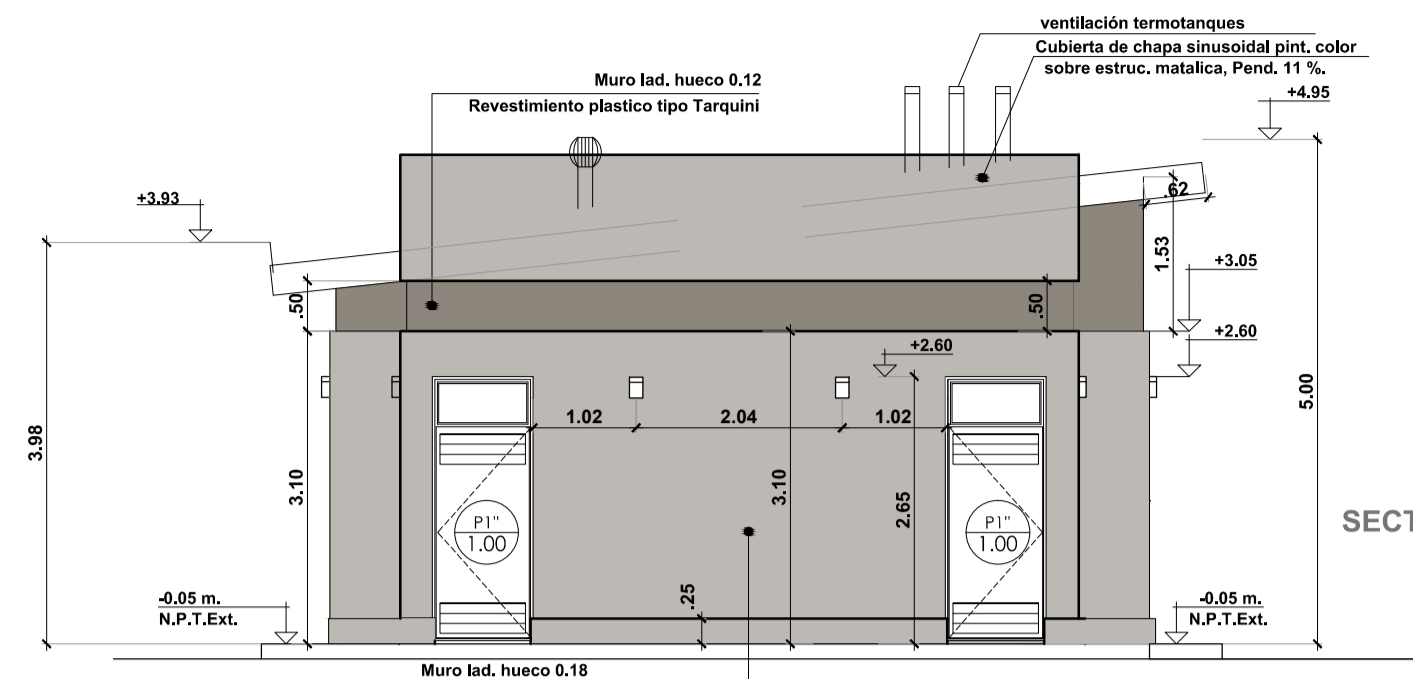
VISTA LATERAL EDIF. B (VEST. PILETA) DESDE CALLE SERRANO
