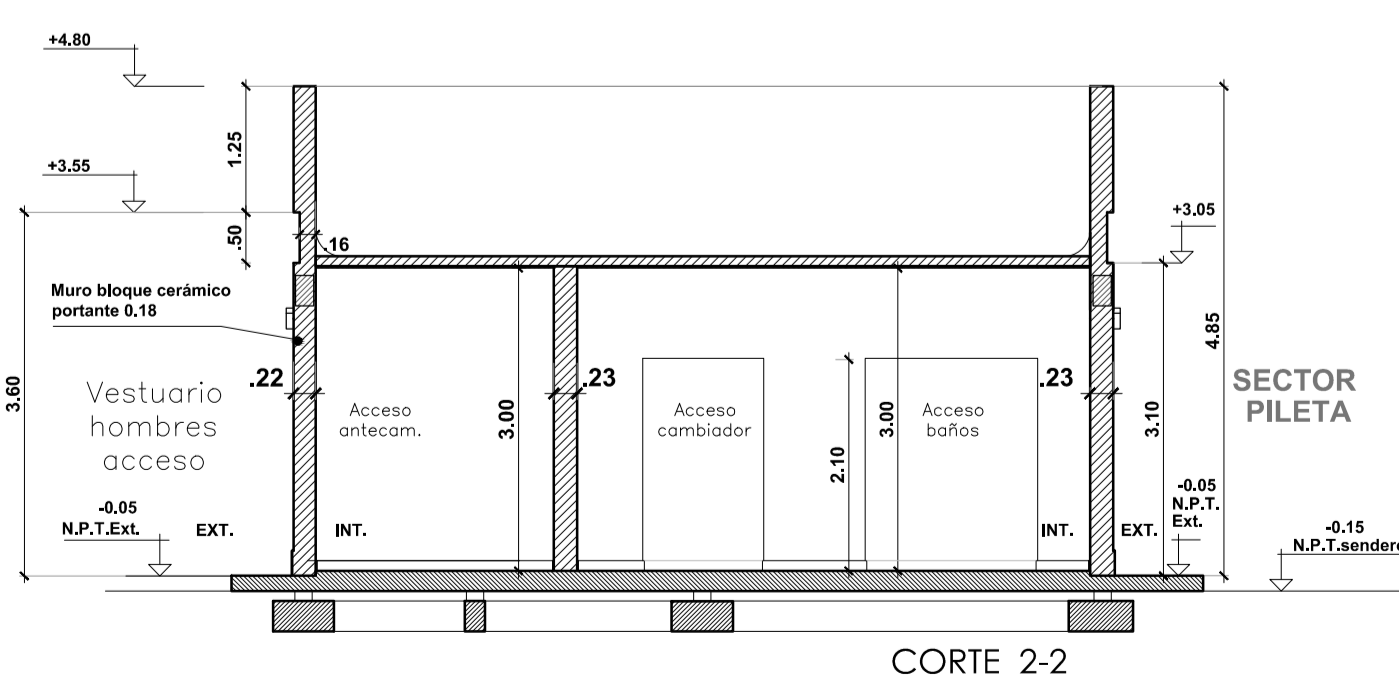
CORTE 2-2
