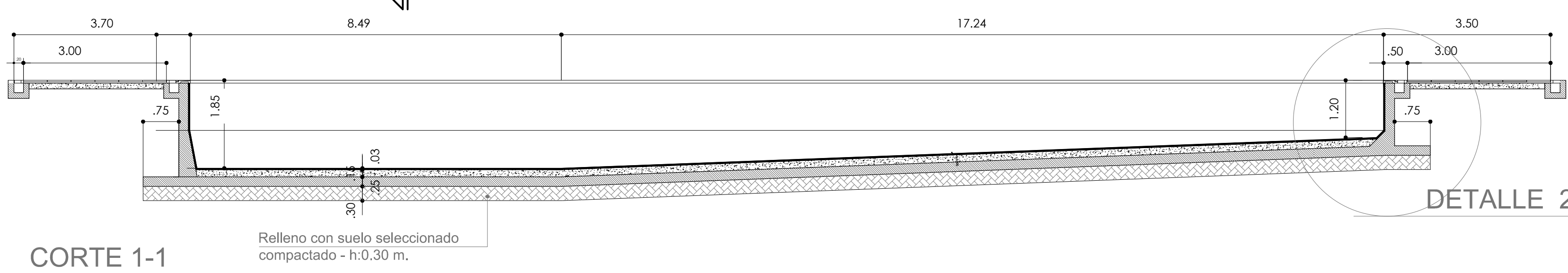
CORTE 1-1
