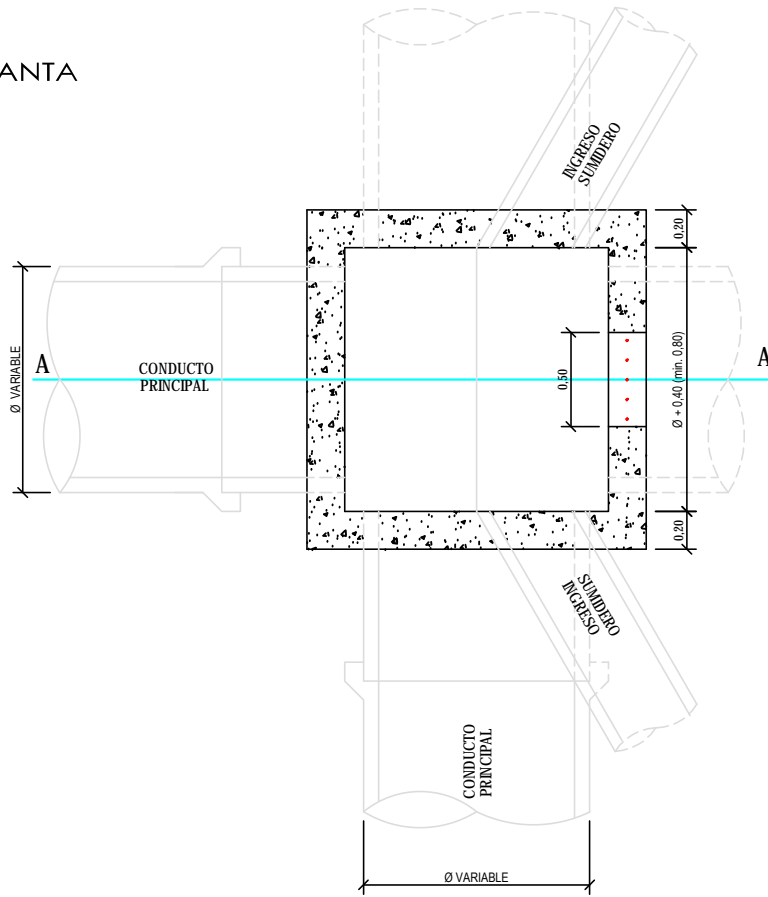
CORTE A-A
