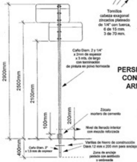
VISTA CONJUNTO ARMADO
