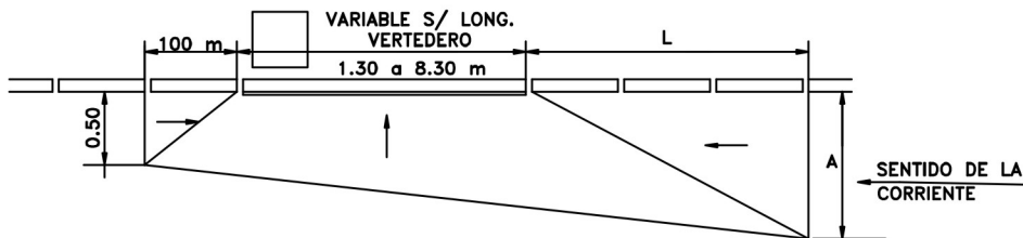
MODIFICACION DE PAVIMENTO PARA FORMACION DE HOYA
