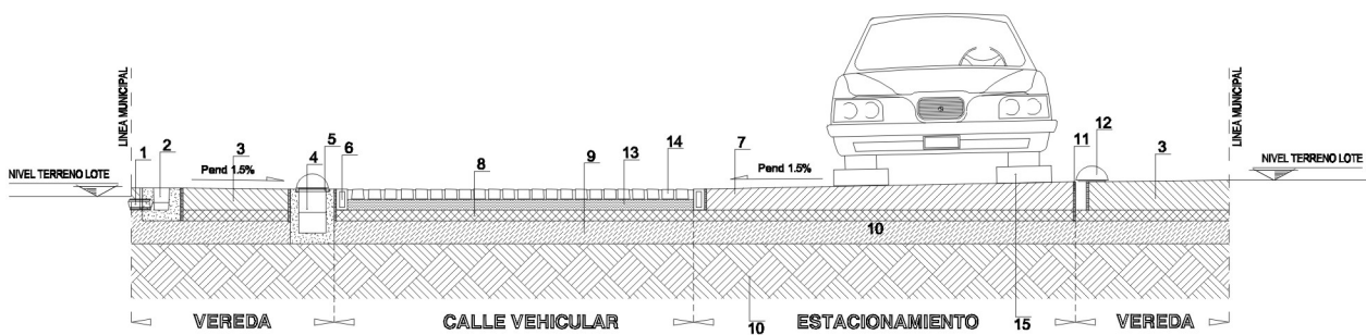
SECCIONESQUEMATICA 2-2
