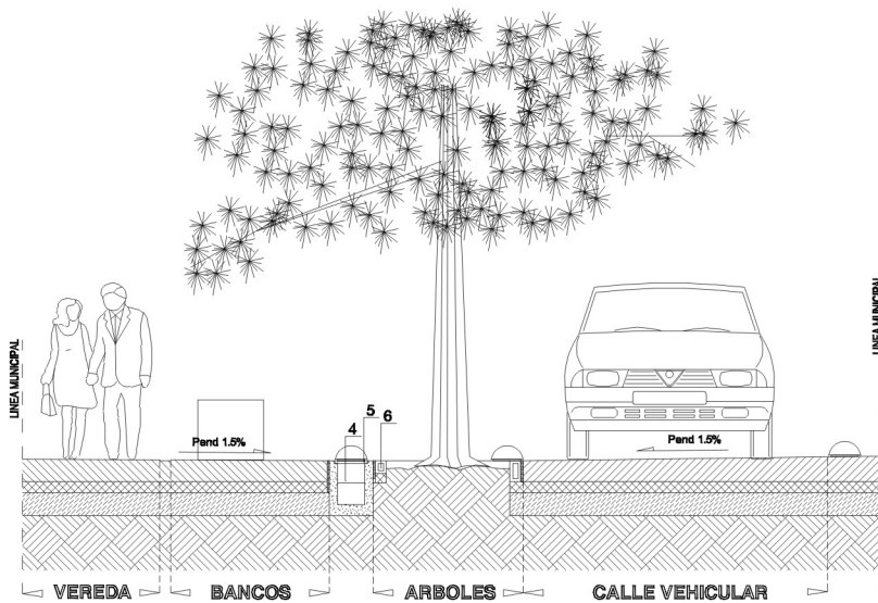
SECCIONESQUEMATICA 3-3
