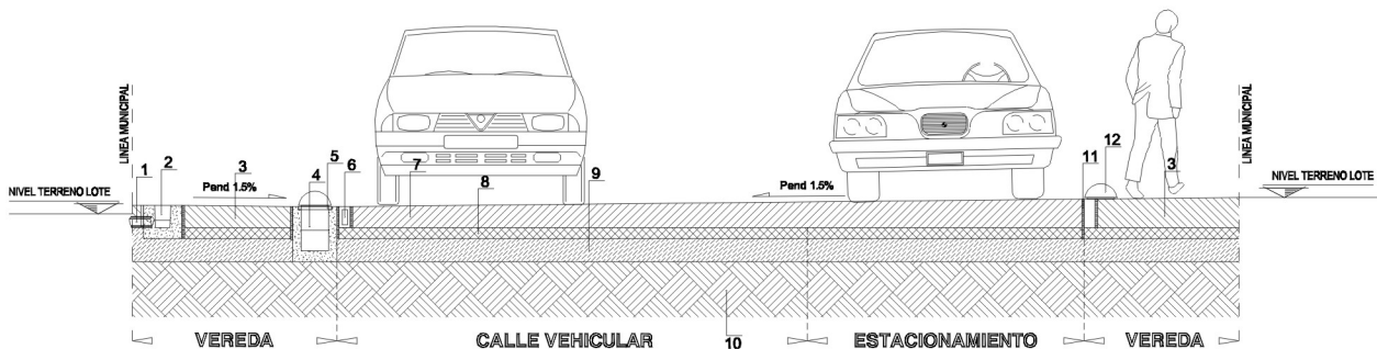
SECCIONESQUEMATICA 1-1
