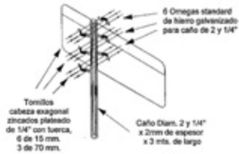
VISTA CONJUNTO ARMADO
