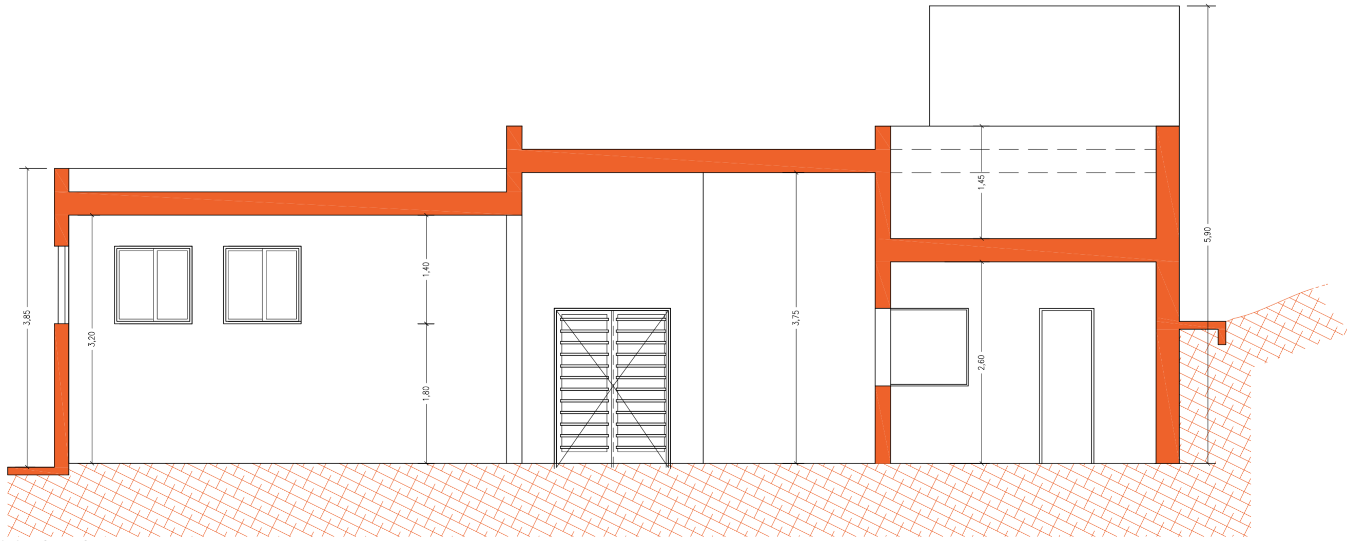
SECCION A_A
