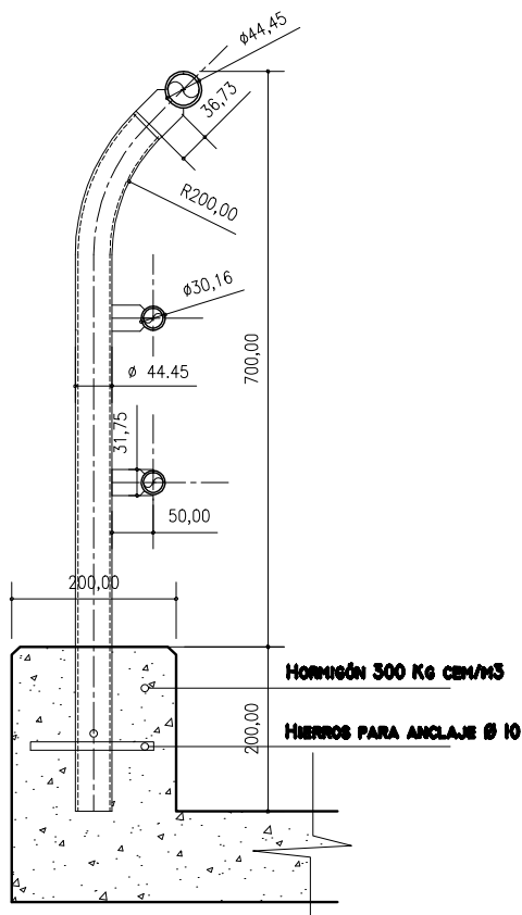
VISTA LATERAL
