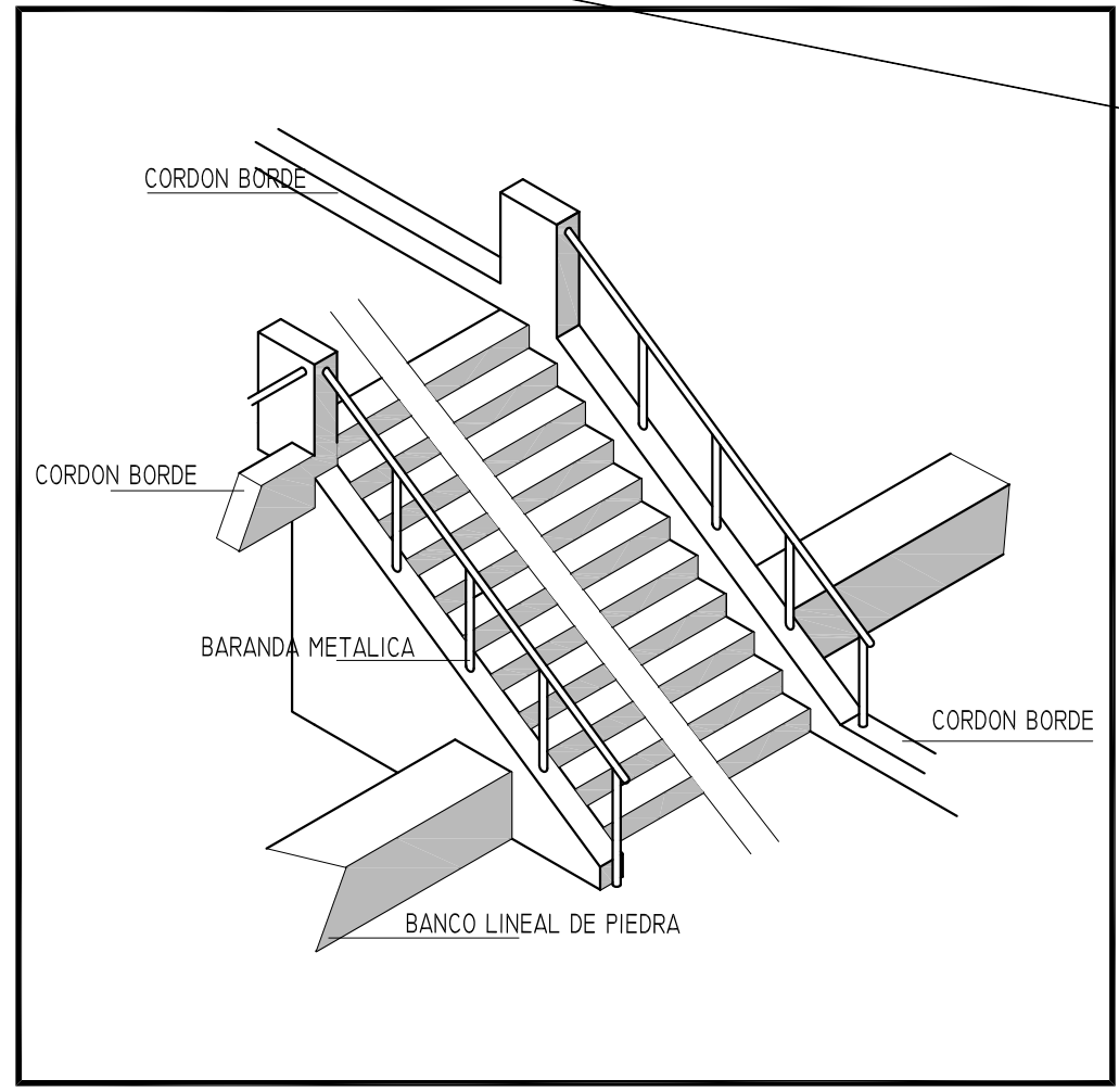
DETALLE ESCALERAS
