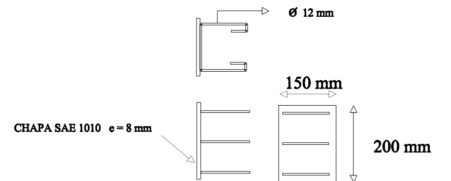
PLACA DE ANCLAJE DE PARANTE DEFENSAS
