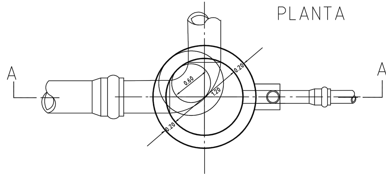
DETALLE A
