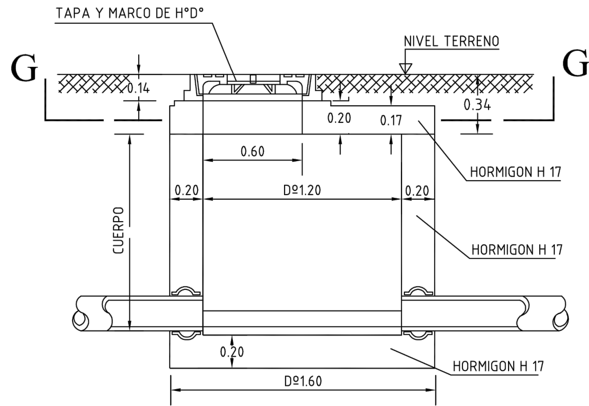
CORTE A-A
