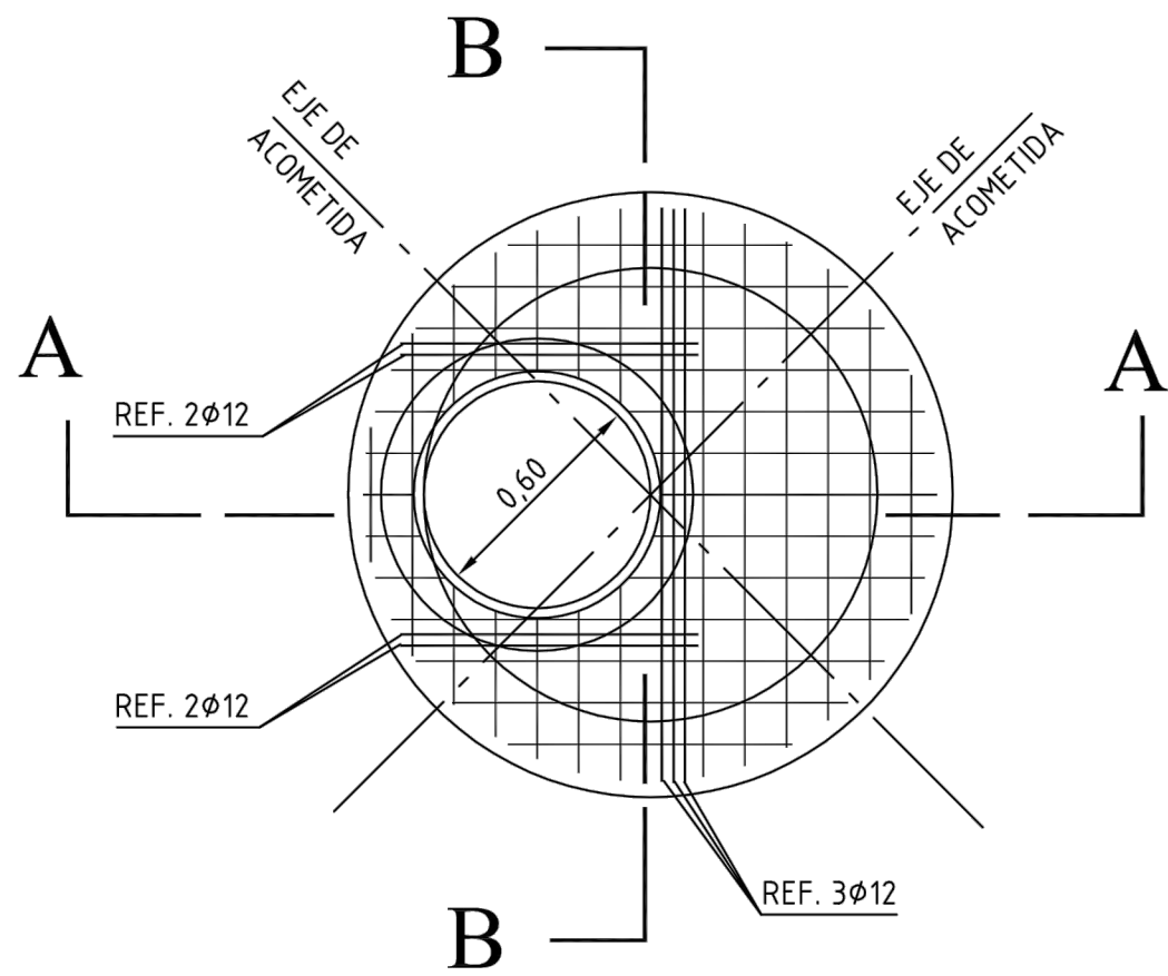
PLANTA POR G-G
