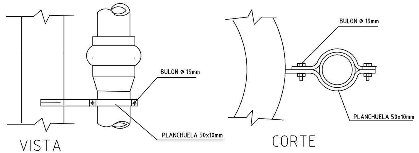
DETALLE A
