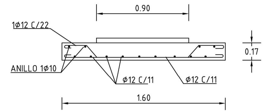
CORTE B-B
