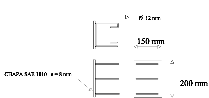
PLACA DE ANCLAJE DE PARANTE BARANDA
