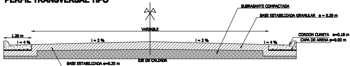
PERFIL TRANSVERSAL TIPO
